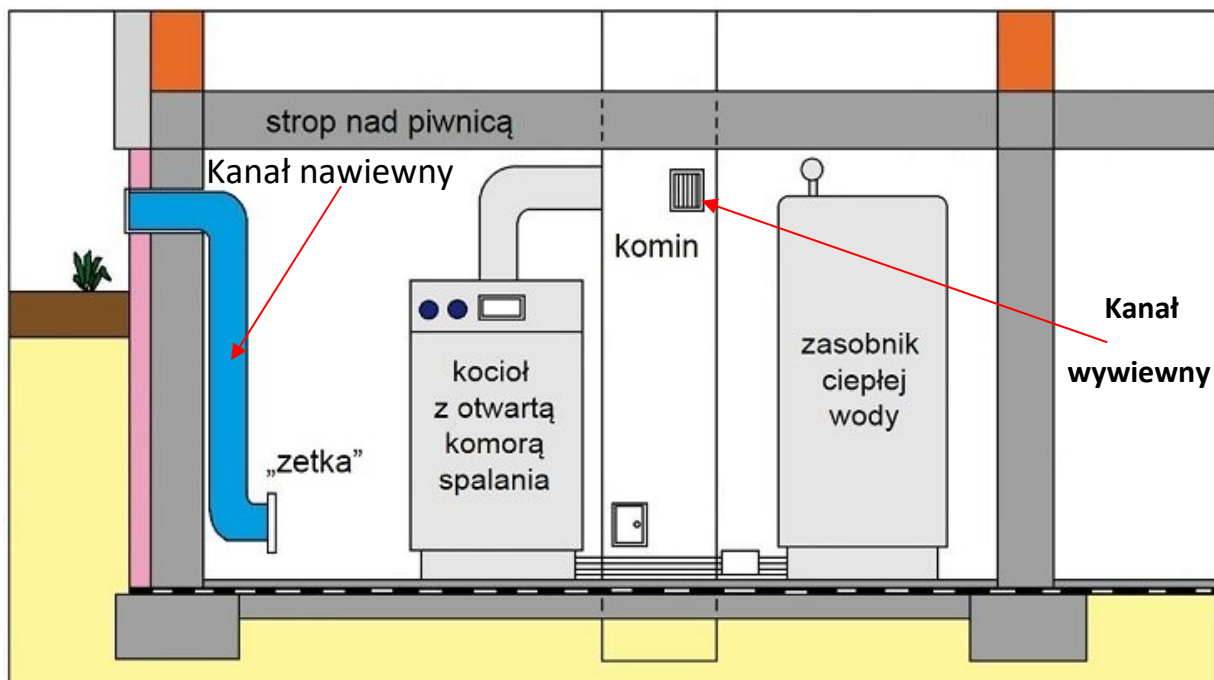
Przykładowy schemat instalacji nawiewno-wywiewnej kotłowni
